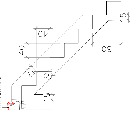
CORTE AA'
