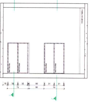
VISTA 4 - INTERNA
