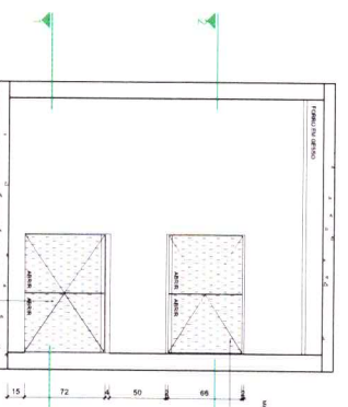
VISTA 4 - EXTERNA
